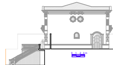
Elevation 04
