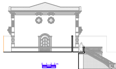
Elevation 02
